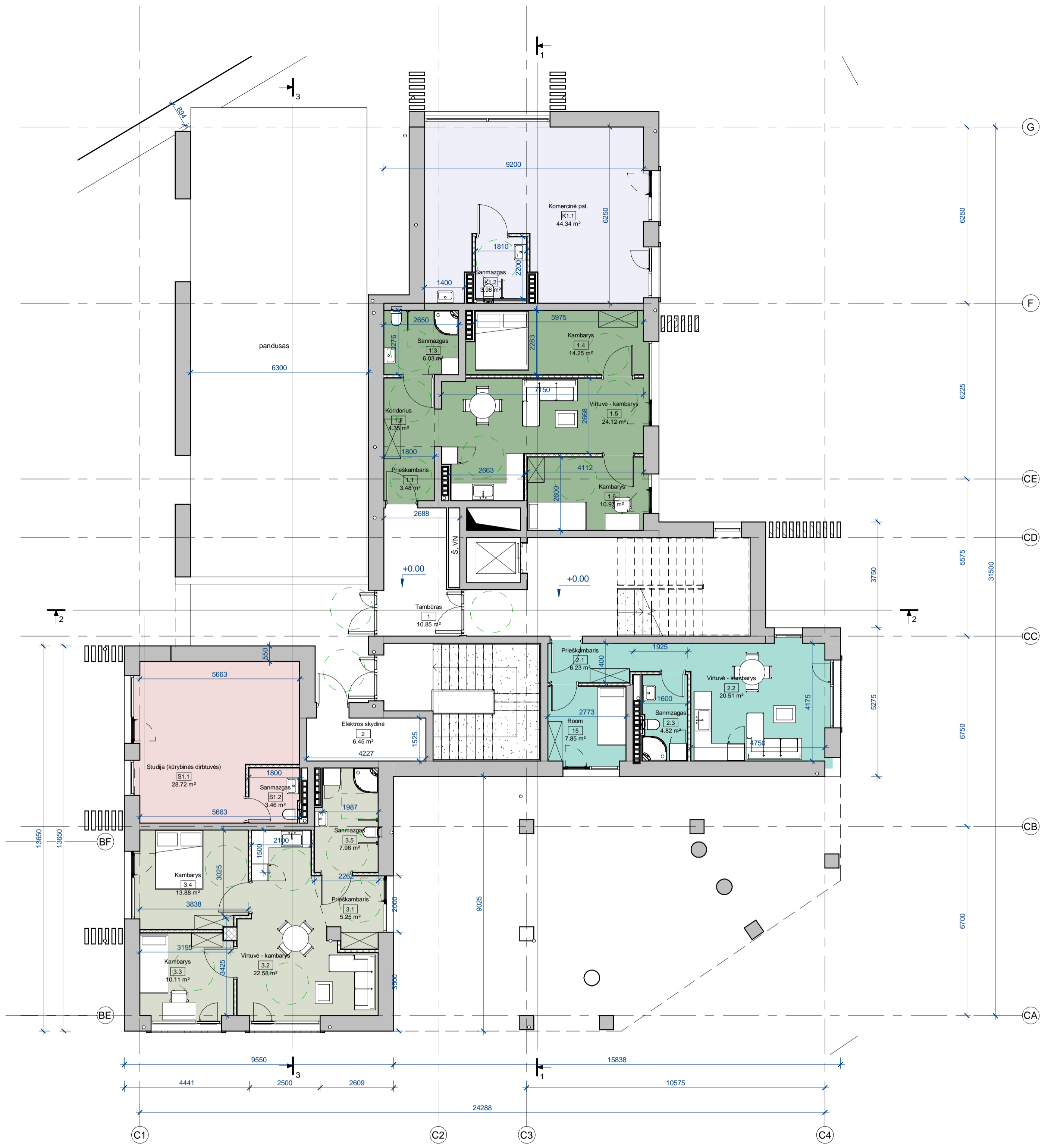
Pirmo aukšto planas 1 : 100
