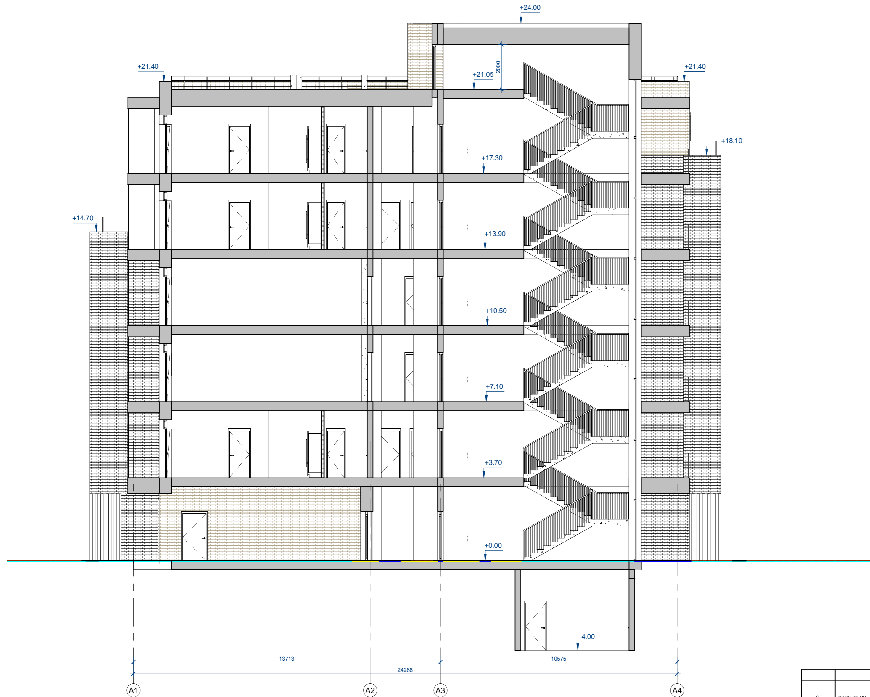
Pjūvis 2-2 1 : 100
