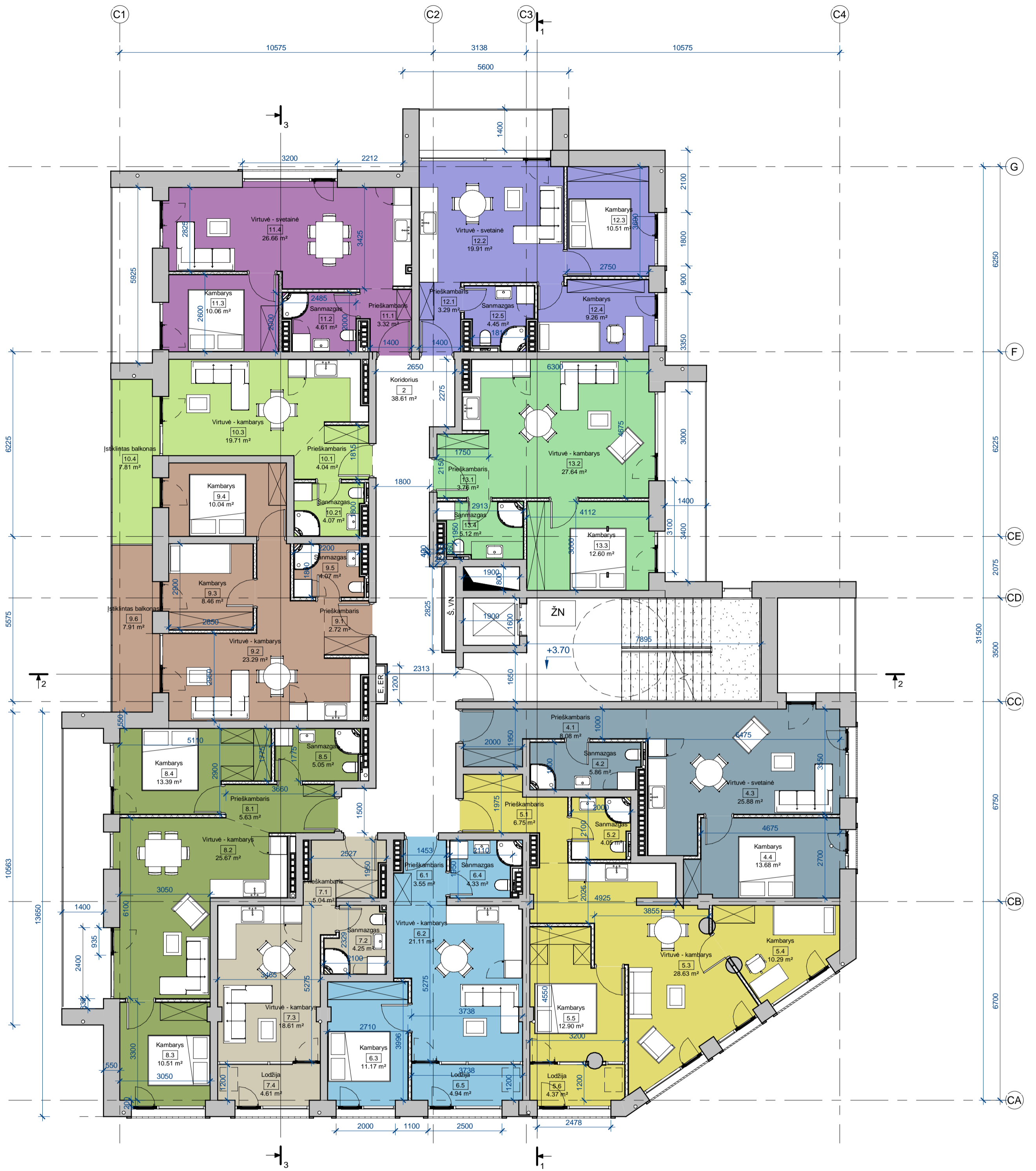
Antro aukšto planas
