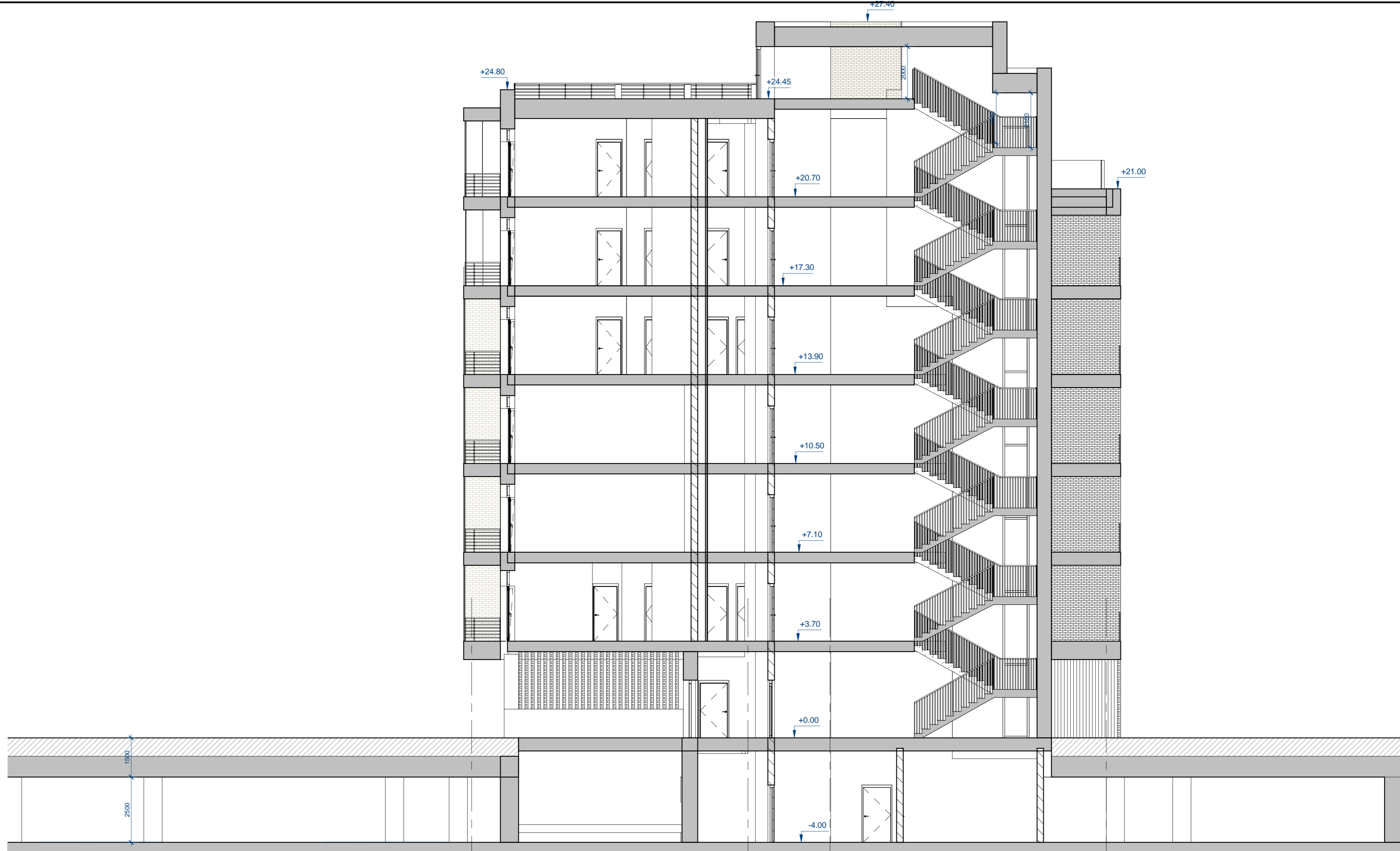
Pjūvis 2-2 1 : 100
