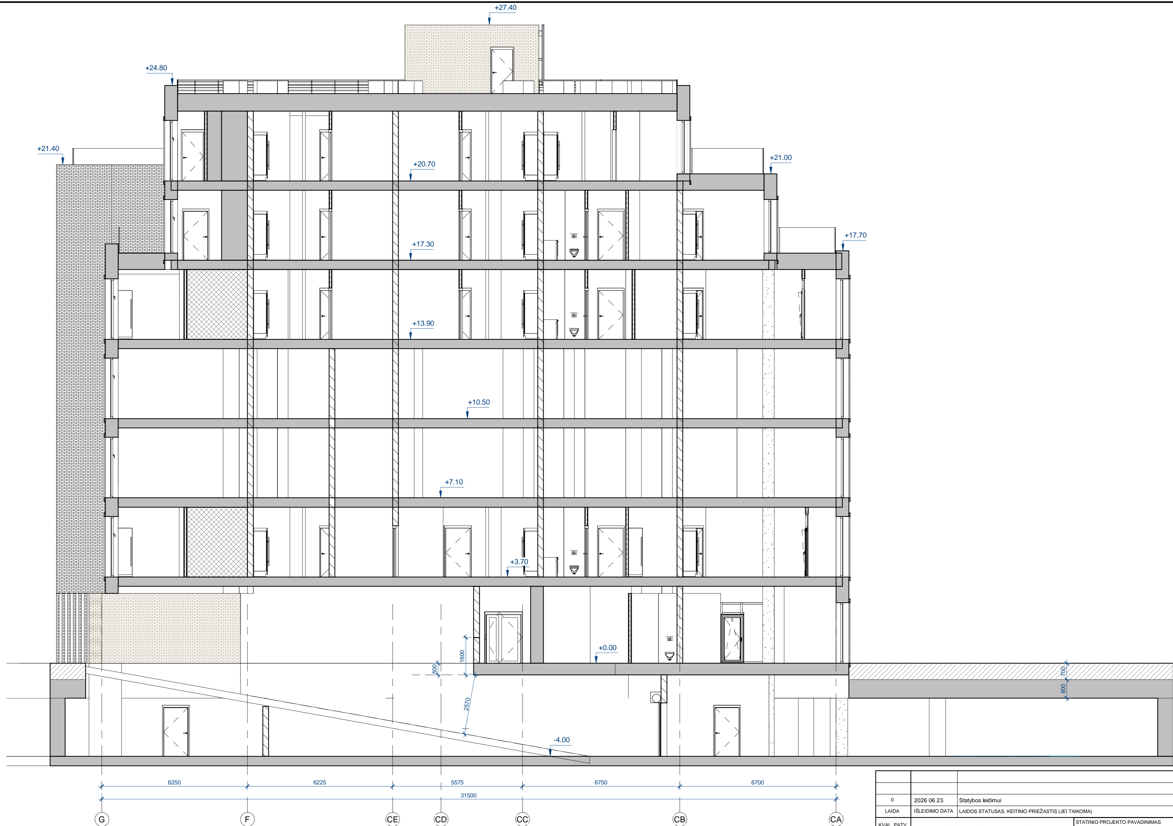
Pjūvis 3-3 1 : 100
