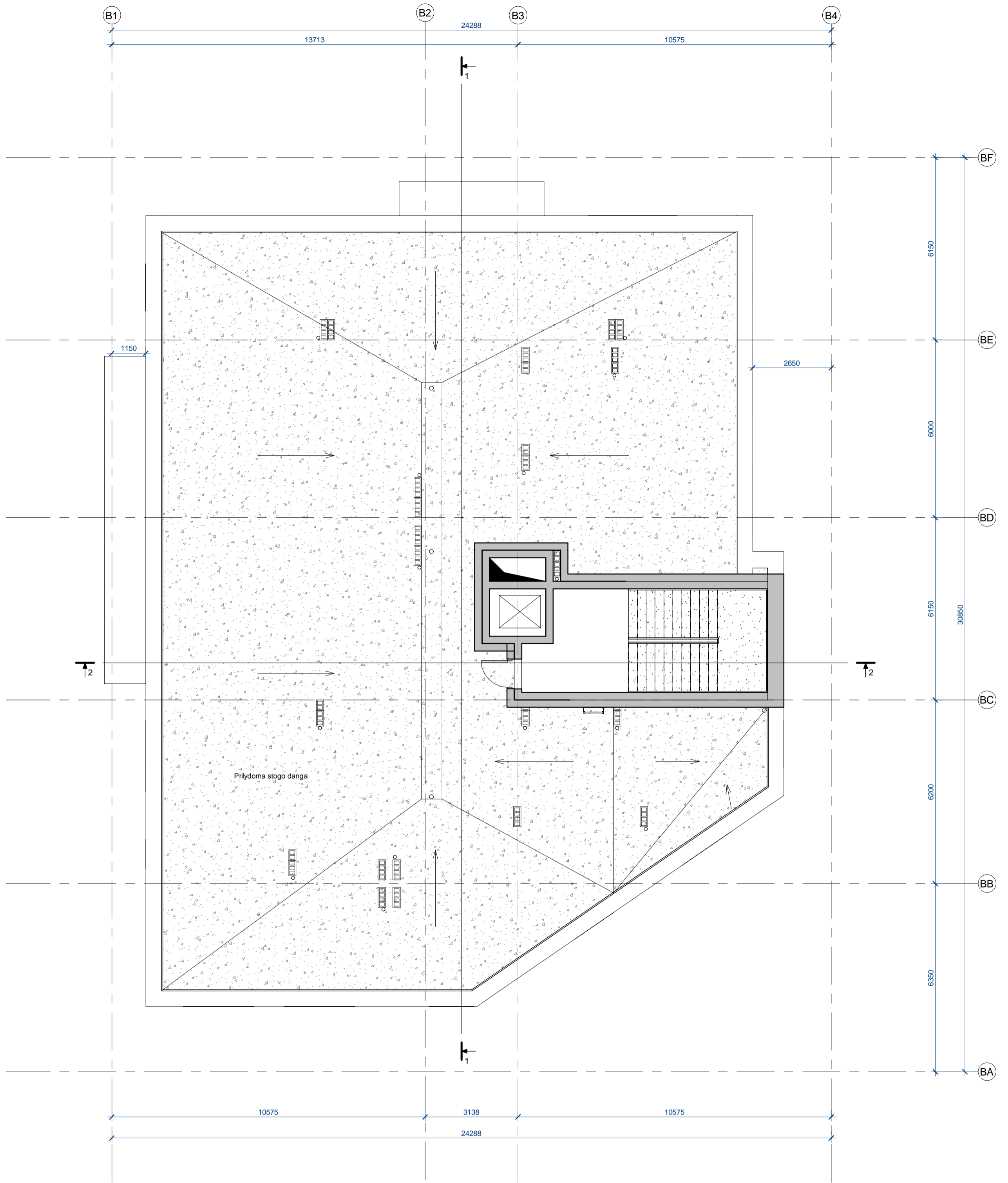
Stogo planas
