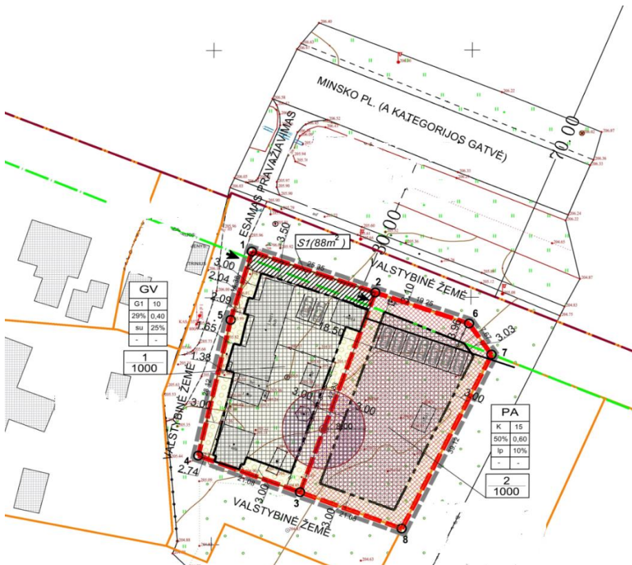
11 pav. Žemės sklypo (kad. Nr. 4162/0100:1068), esančio Vilniaus r. sav., Nemėžio sen., Kuprioniškių k., Minsko pl. 53, detaliojo plano rengimas. Pagrindinis brėžinys (Rengiamas)
