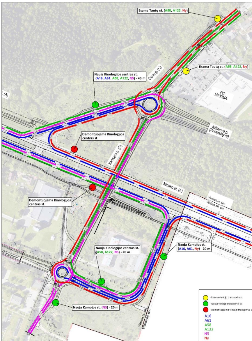
17 pav. Viešasis transportas Kamojos g. – Gurių g. mazgas
