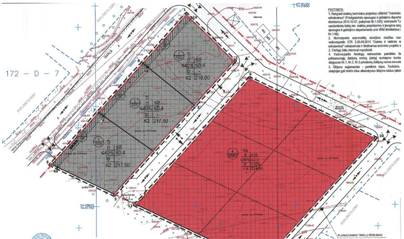
9 pav. Apie 12 ha teritorijos prie Gurių gatvės detaliojo plano (registro Nr. 78016) keitimas sklypuose Moravų g. 1, 3, 5, 7, 9, 11, 13, 15 ir 17. Pagrindinis brėžinys.
