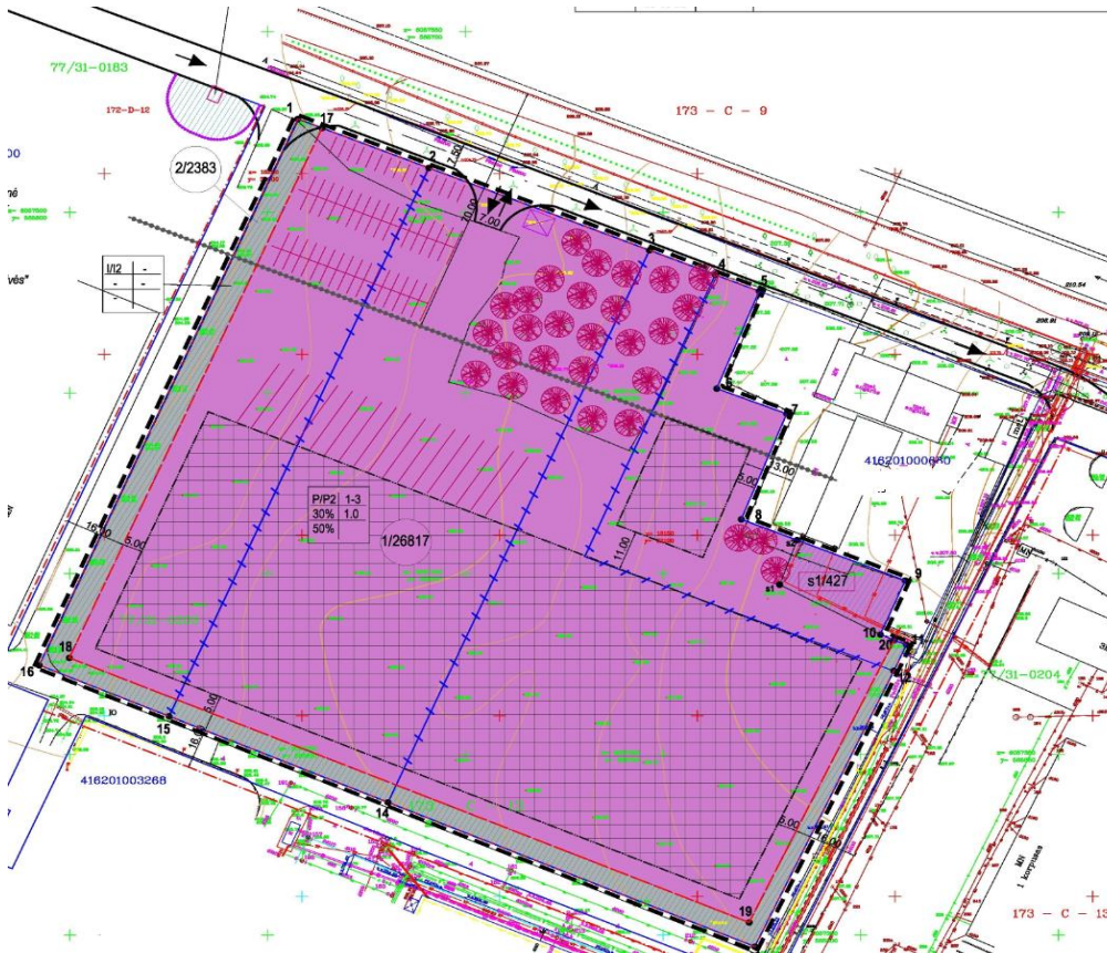
10 pav. Žemės sklypų (kad. Nr. 4162/0100:705, 4162/0100:704, 4162/0100:685, 4162/0100:684), Kuprioniškių k., Nemėžio sen., Vilniaus r. Detalusis planas. Pagrindinis brėžinys.
