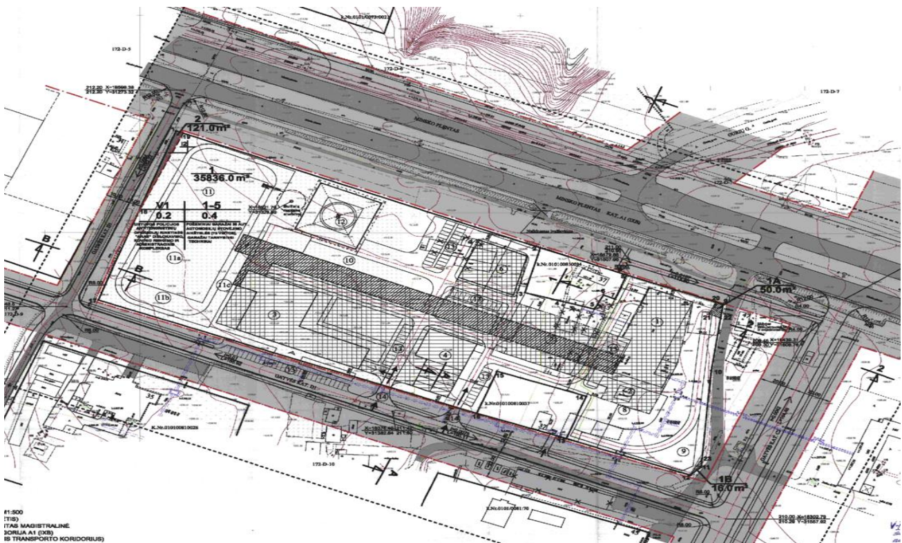
7 pav. Žemės sklypo (Kad. Nr. 0101/0081:63) Minsko pl. 37, Vilniuje, detalusis planas. Pagrindinis brėžinys.
