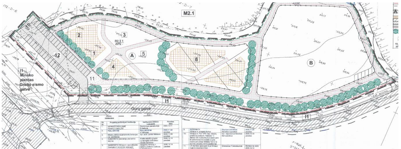
8 pav. Teritorijos prie Minsko plento nedidelių veiklos mastų detalus planas. Pagrindinis brėžinys.
