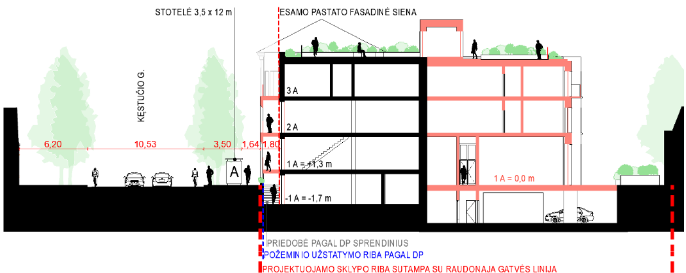
Nr.8. Schema - pjūvis per Kęstučio gatvę ir rekonstruojamą pastą.
