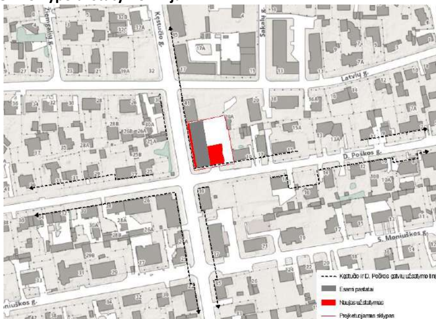
Nr.7. Schema Kęstučio ir D. Poškos gatvių užstatymo linija.
