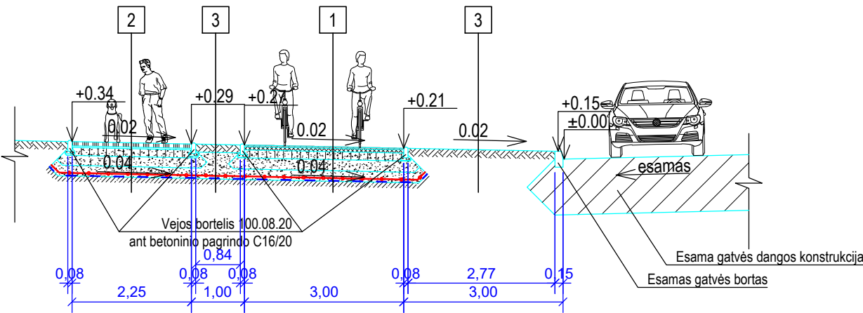
PJŪVIS 1-1 M1:100
