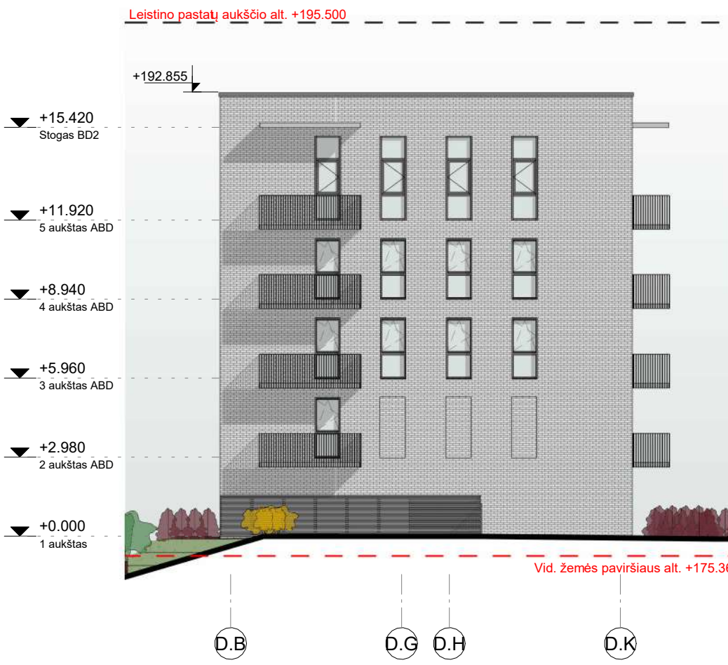
3. FASADAS TARP AŠIŲ D.B - D.K (Kiemo fasadas šalia kotedžo) 1 : 200
