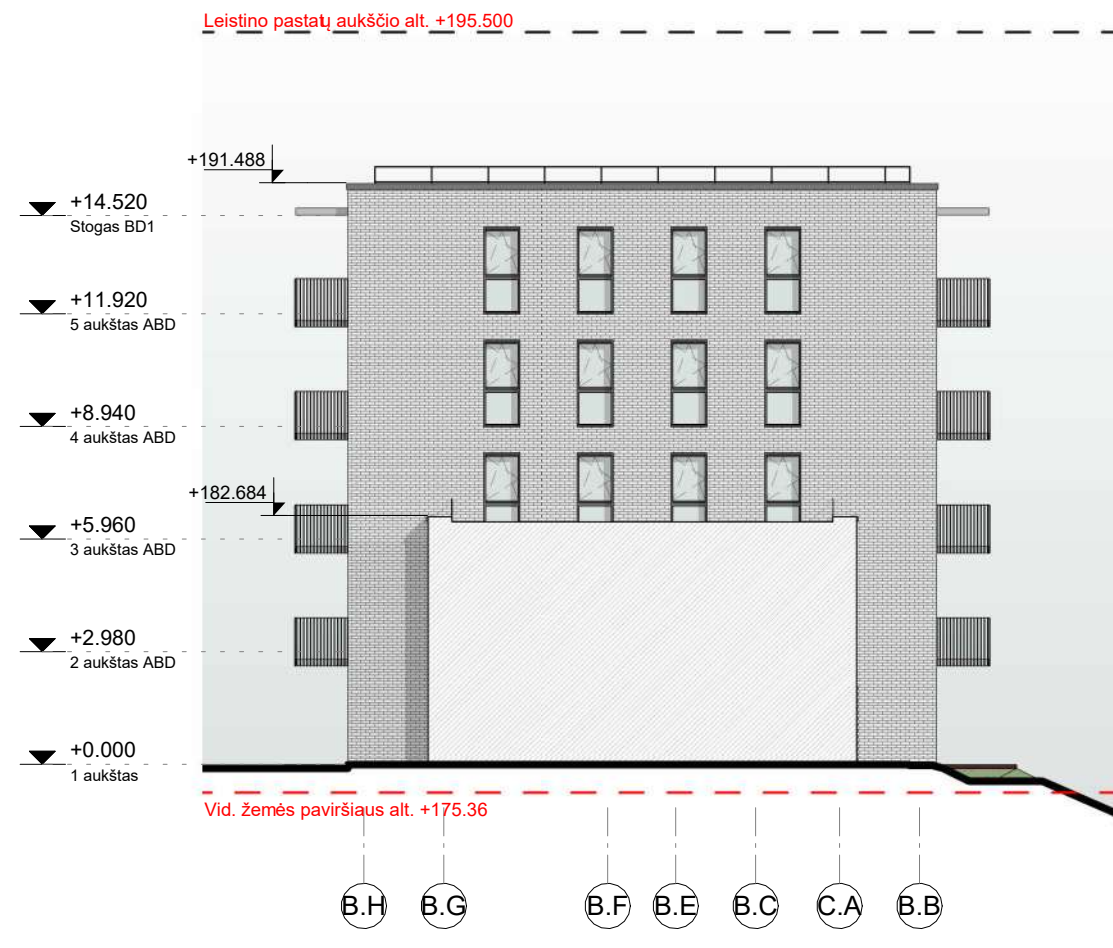
4. FASADAS TARP AŠIŲ B.H - B.B (Kiemo fasadas šalia kotedžo) 1 : 200
