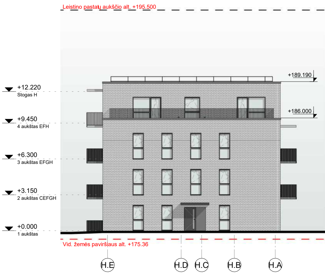
18. FASADAS TARP AŠIŲ H.E - H.A (Kiemas fasadas su įėjimu) 1 : 200
