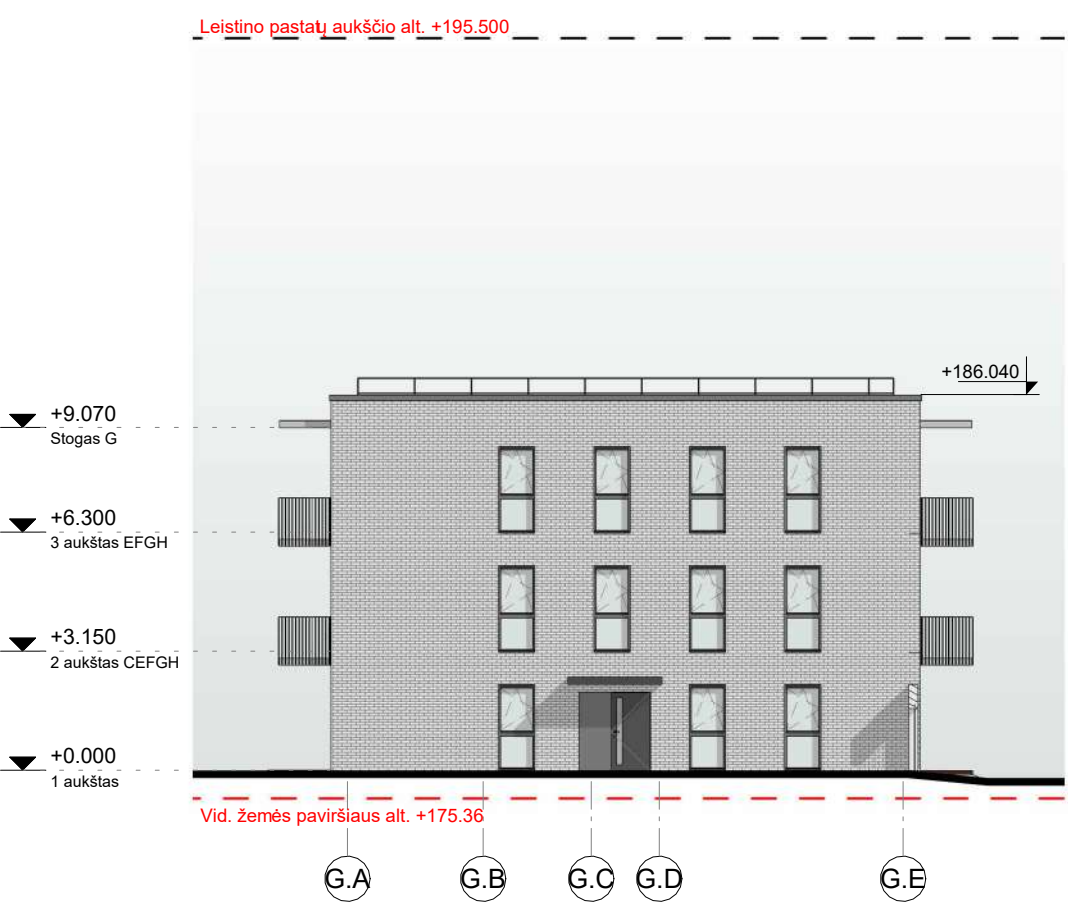
19. FASADAS TARP AŠIŲ G.A - G.E (Kiemas fasadas su įėjimu) 1 : 200
