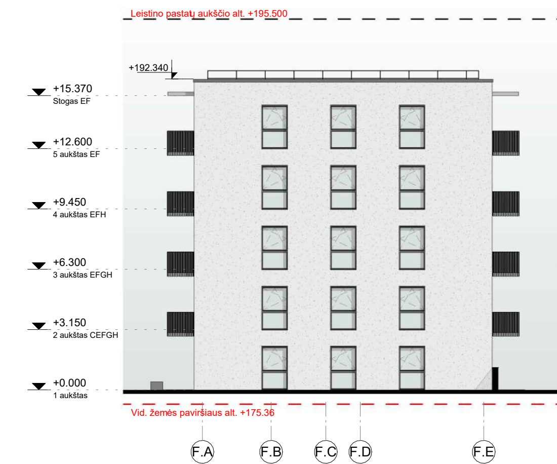
14. FASADAS TARP AŠIŲ F.A - F.E (Kiemas fasadas) 1: 200
