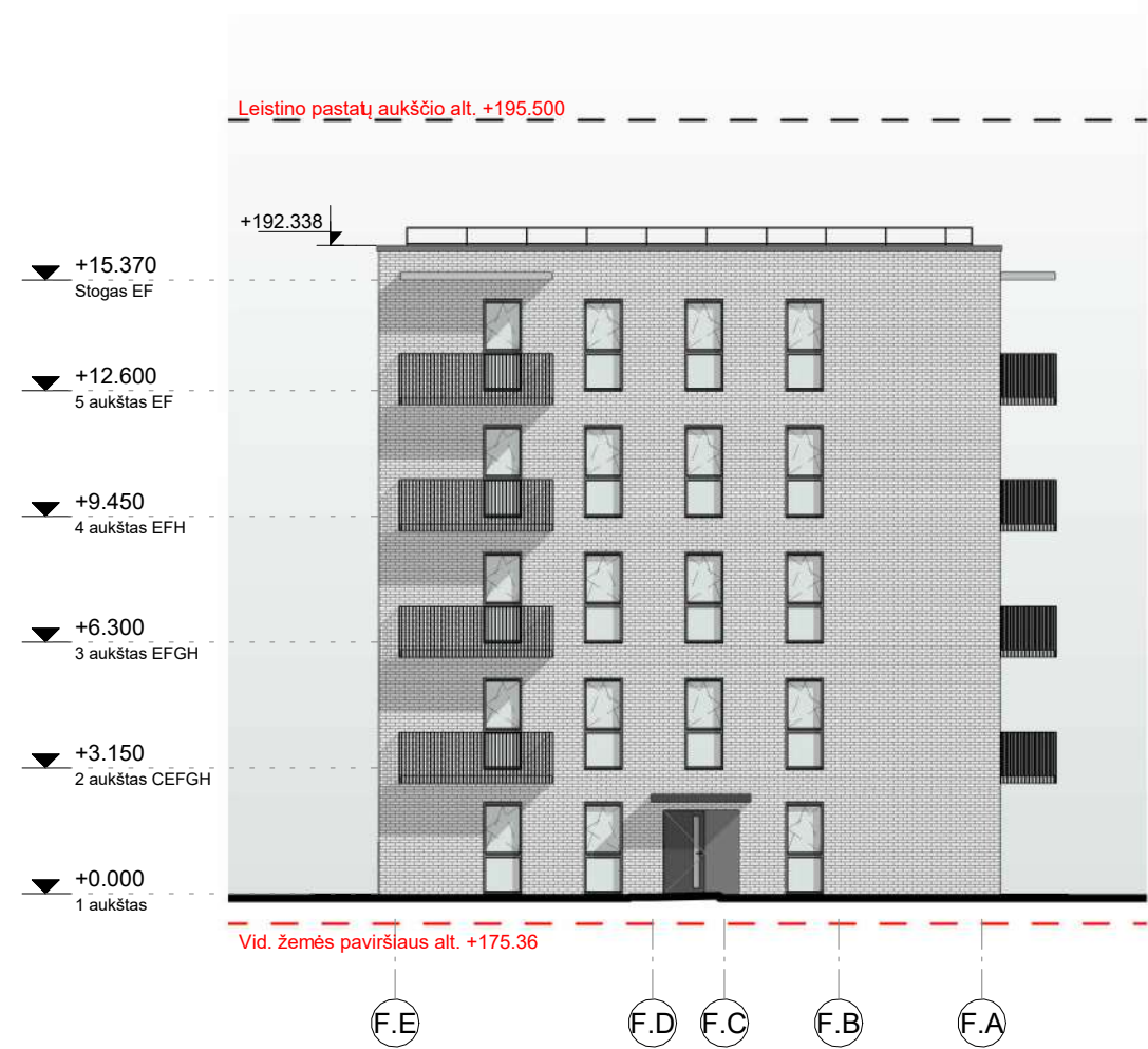
12. FASADAS TARP AŠIŲ F.E - F.A (Kiemas fasadas su įėjimu) 1: 200
