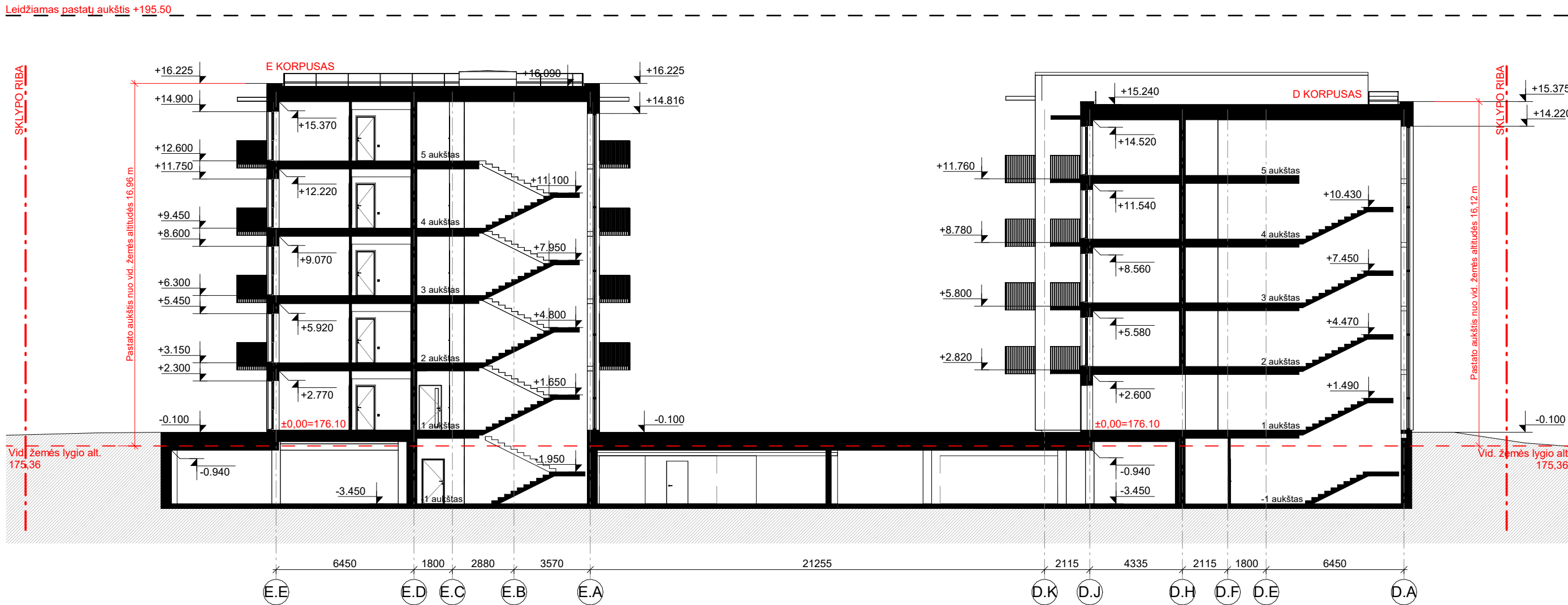
4. PJŪVIS TARP AŠIŲ E.E - D.A 1 : 200
