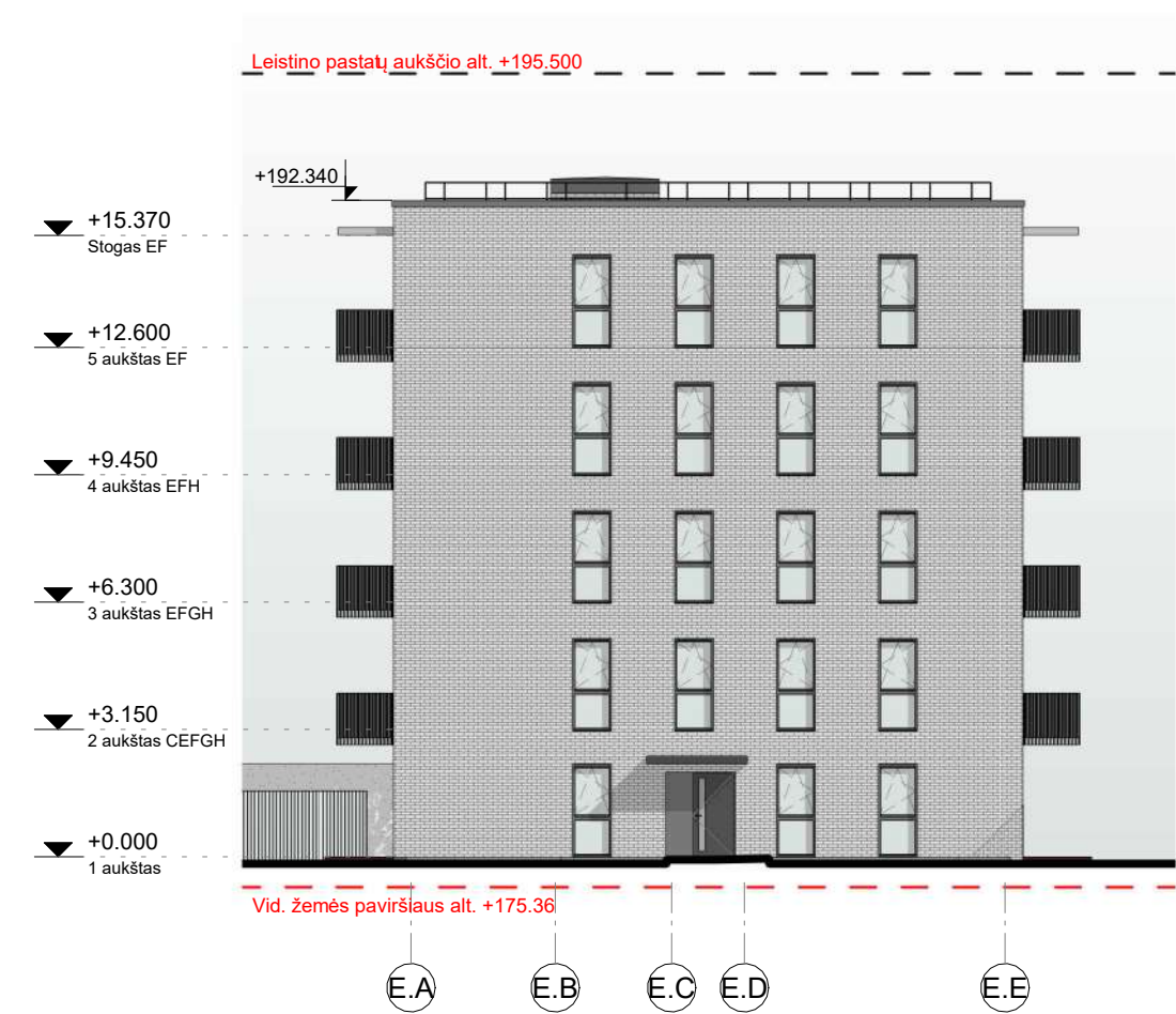
11. FASADAS TARP AŠIŲ E.A - E.E (Kiemas fasadas su įėjimu) 1: 200
