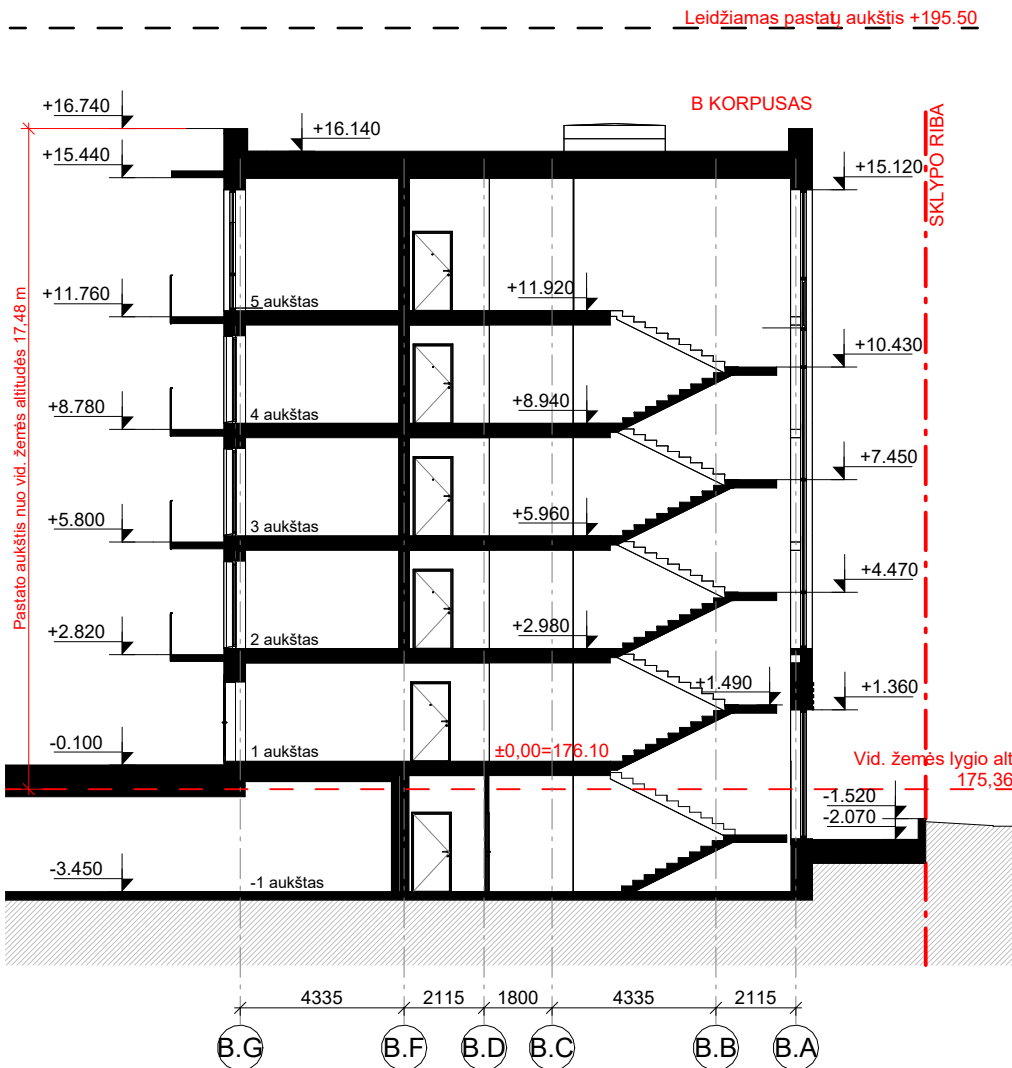
Pjūvis 2 - 2 1 : 200
