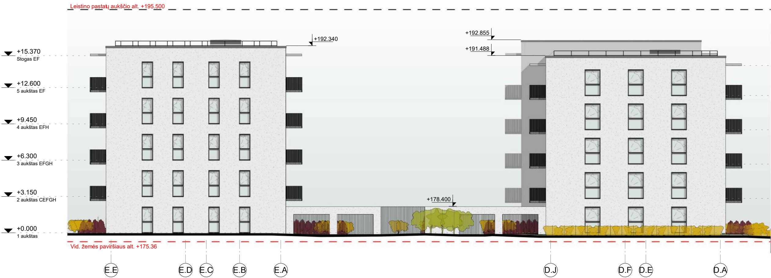
9. FASADAS TARP AŠIŲ D.A - E.E (Pietinis fasadas šalia daugiabučio) 1: 200
