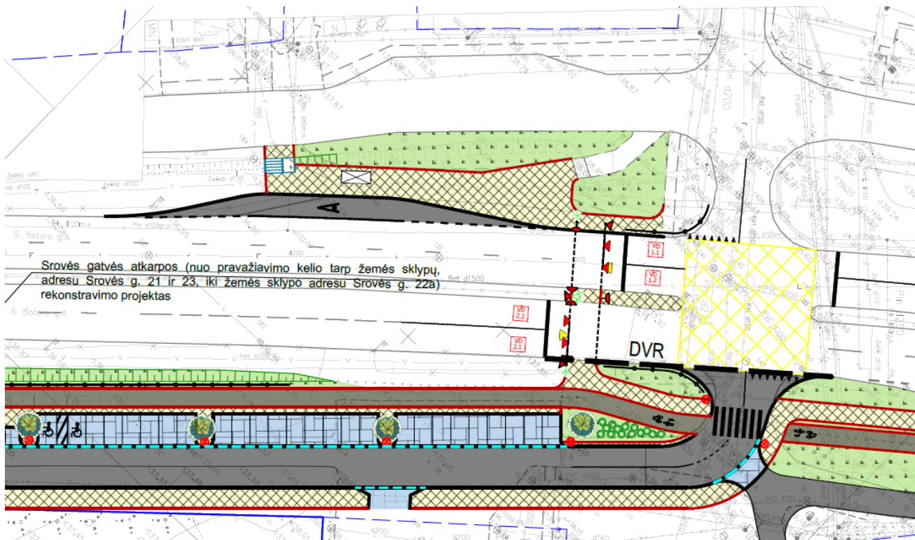
2 pav. Reguluojamos sankryžos planiniai sprendimai
