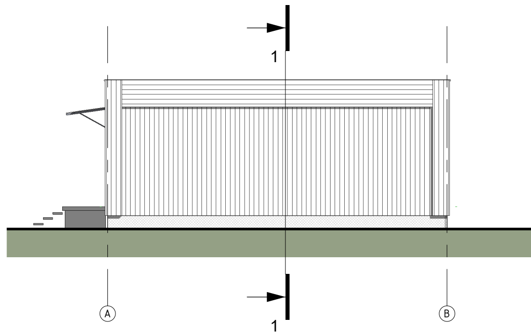
FASADAS TARP AŠIŲ A-B 1 : 100
