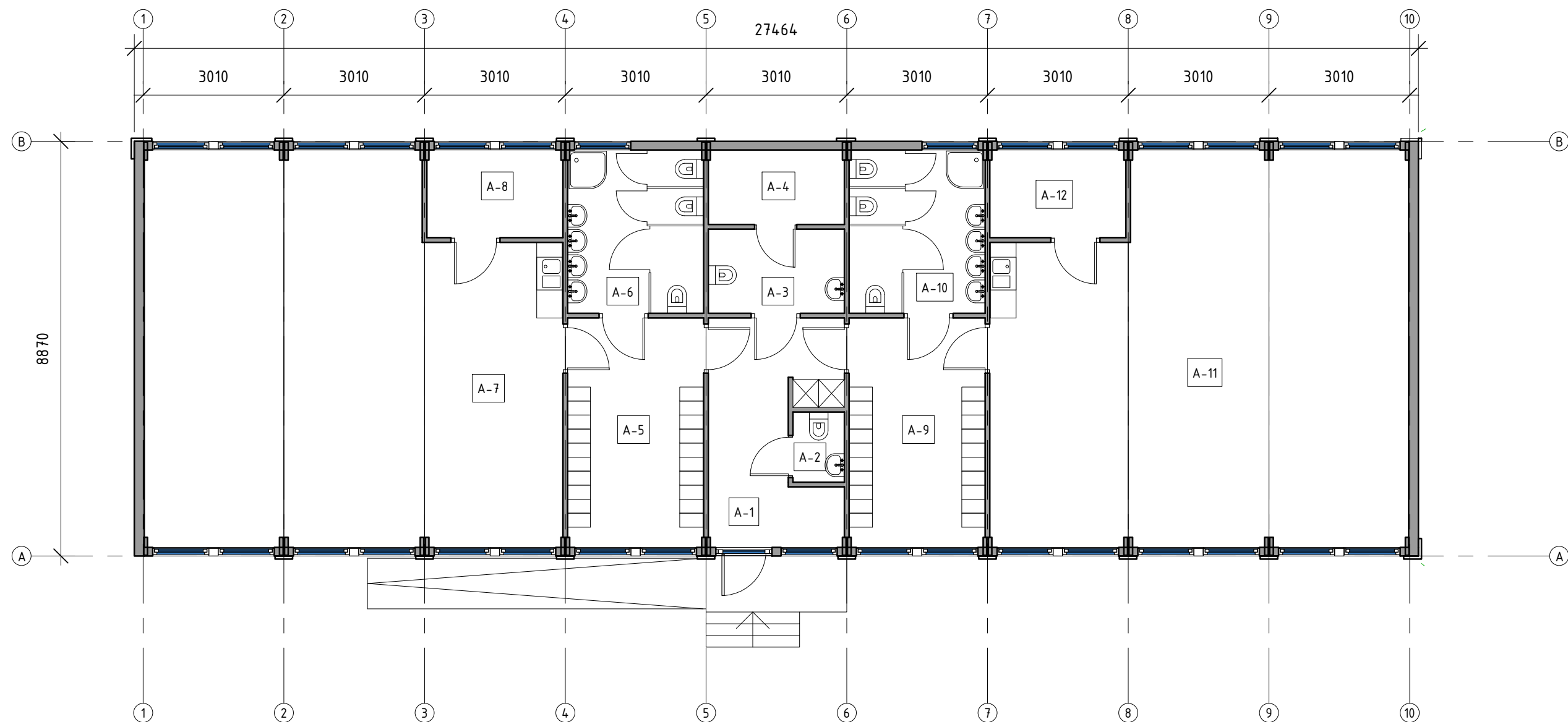
PLANAS 1 : 100
