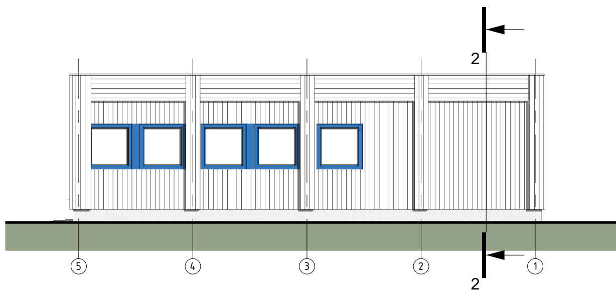
FASADAS TARP AŠIŲ 5-1 1 : 100
