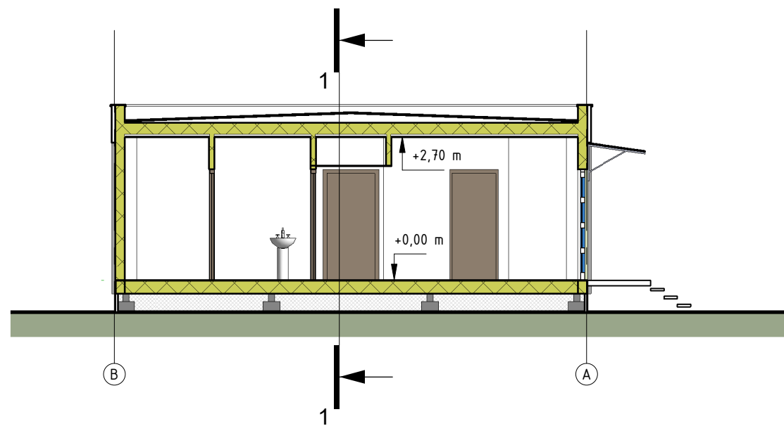
PJŪVIS 2-2 1 : 100
