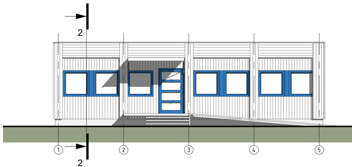
FASADAS TARP AŠIŲ 1-5 1 : 100
