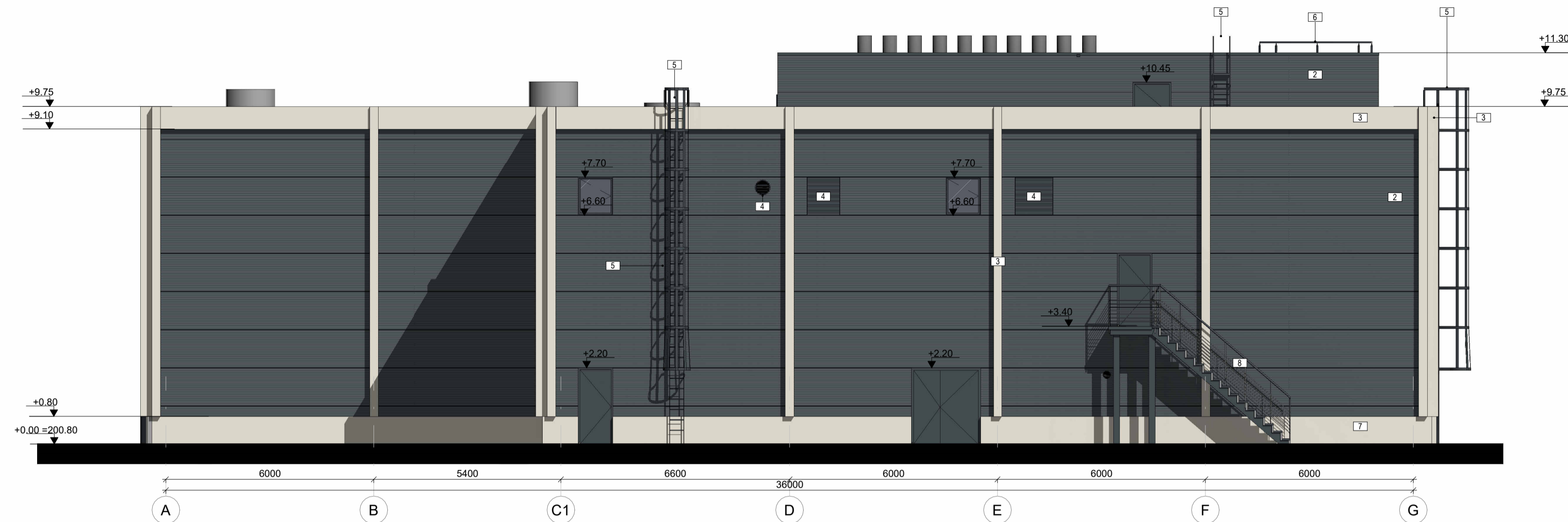
Fasadas tarp ašiu A-G 1:100
