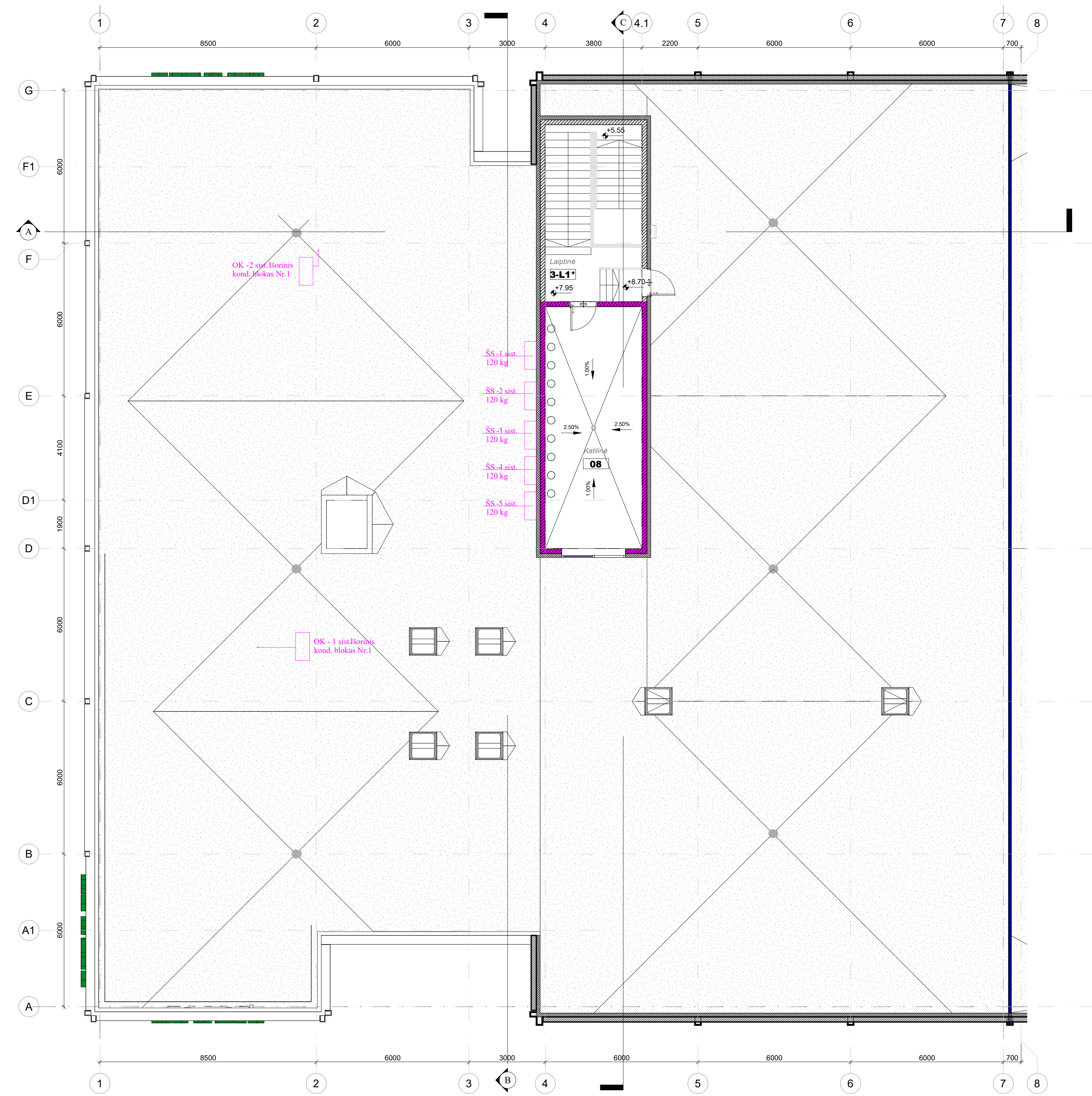
ANSTATO AUKŠTO PLANAS 1:100
