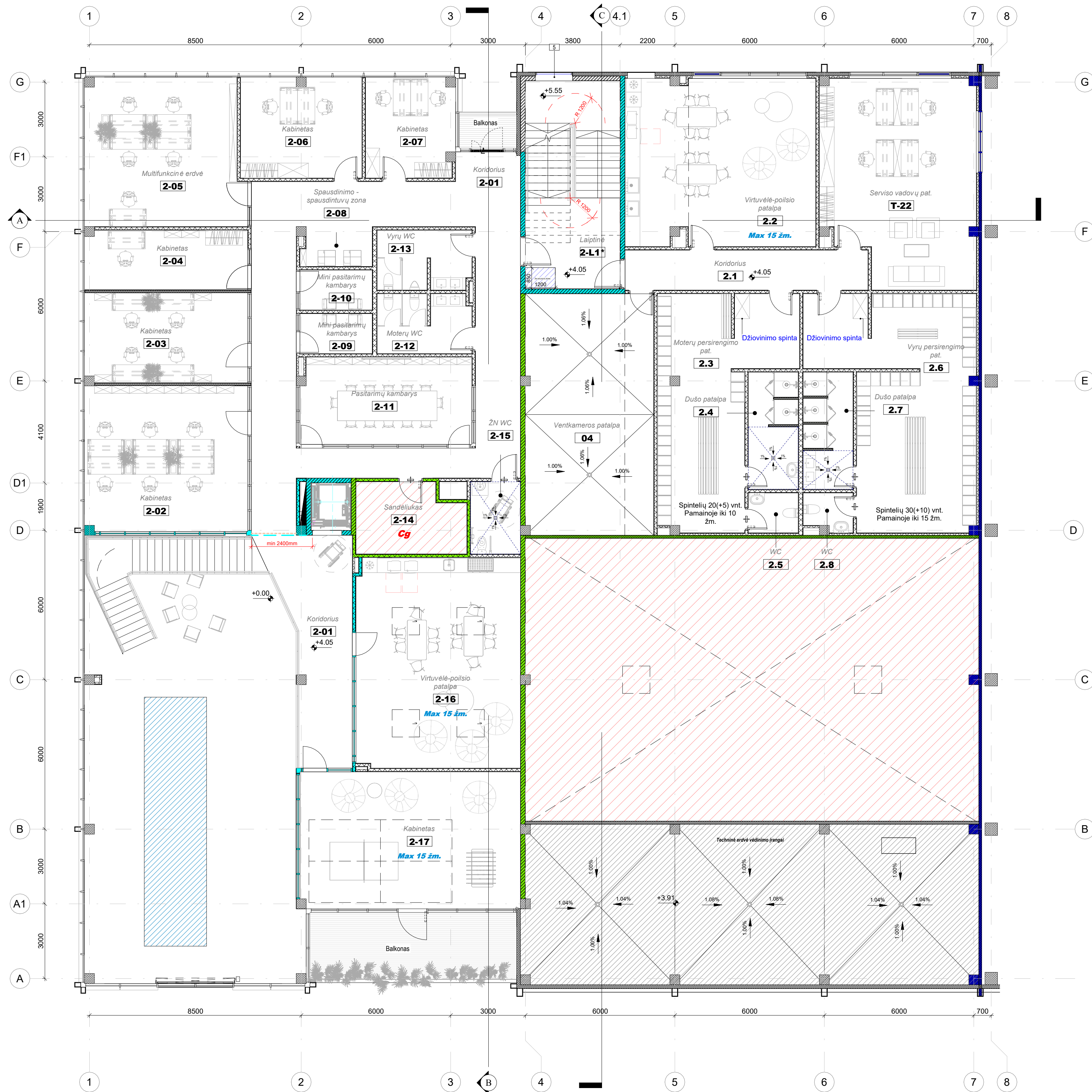
ANTRO AUKŠTO PLANAS 1:100
