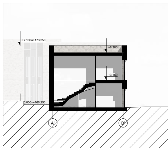
Pjūvis 11-11
